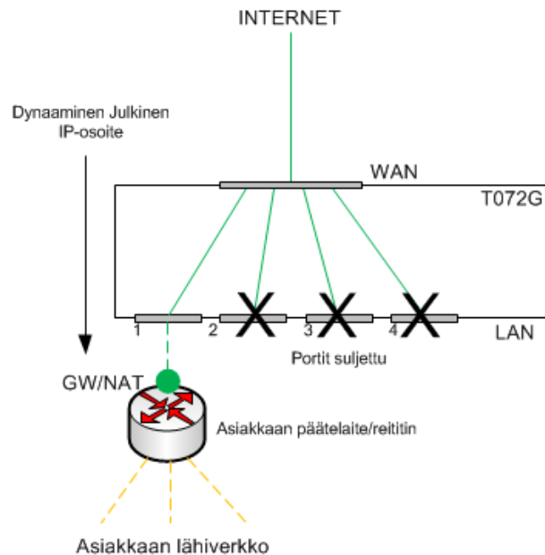
Kuva 5: Päätelaitteen sillattu toimintatila
