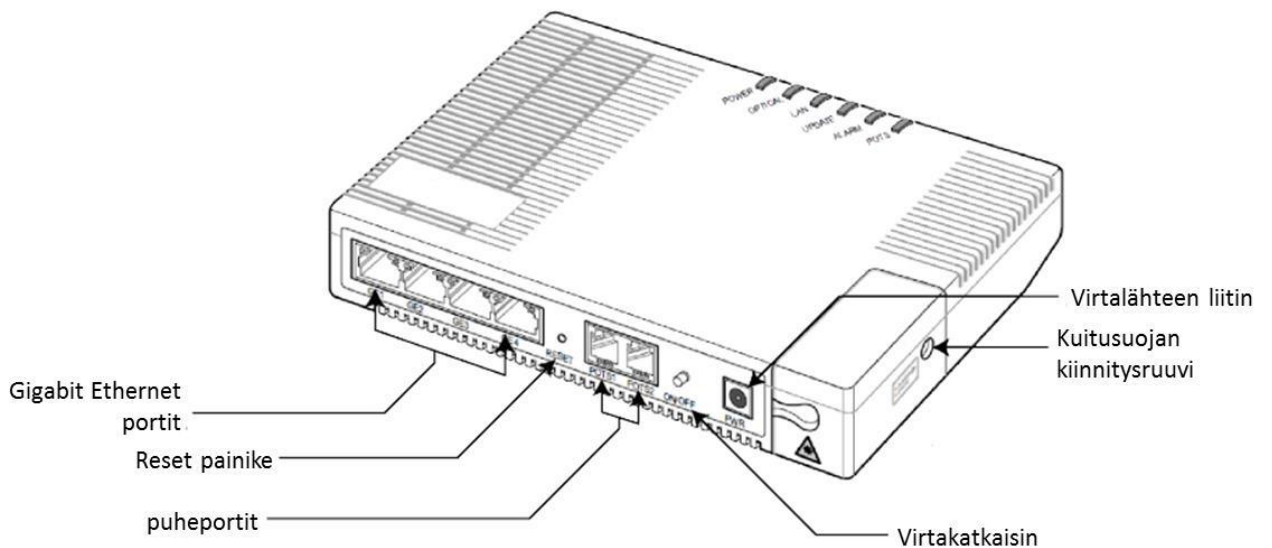
Kuva: päätelaitteen yleiskuva ja liitännät
