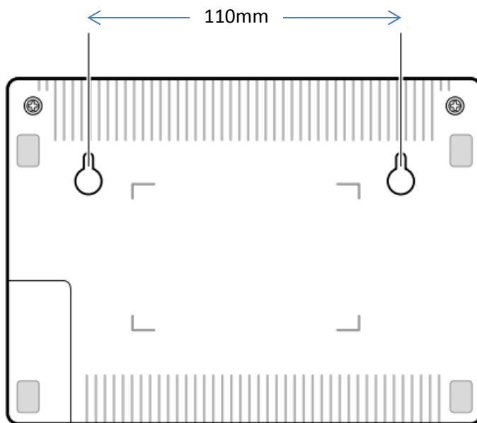
Kuva: Päätelaitteen ruuvihahlot seinäkiinnitystä varten
