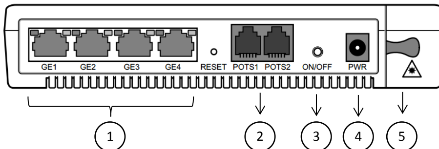
Kuva: päätelaitteen yleiskuva ja liitännät
