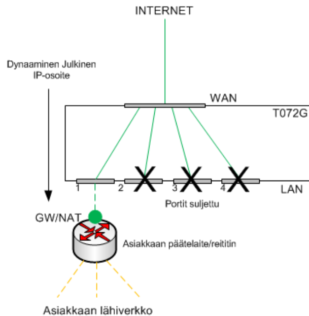
Kuva: Päätelaitteen sillattu toimintatila
