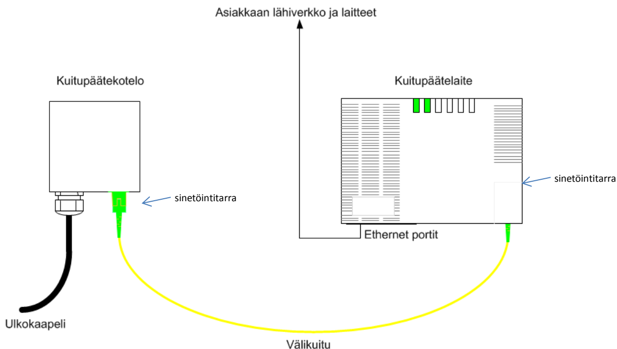
Kuva: Kuitupäätelaite kytkeminen seinälle päätetekotelon läheisyyteen
